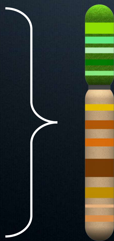
Chromatid
