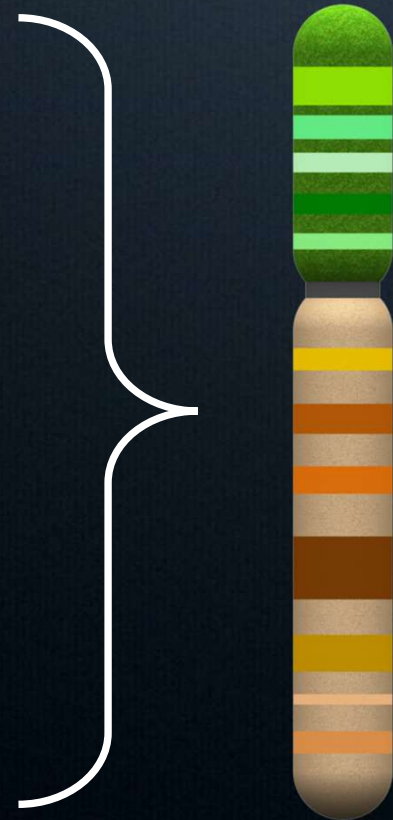
Chromatid
