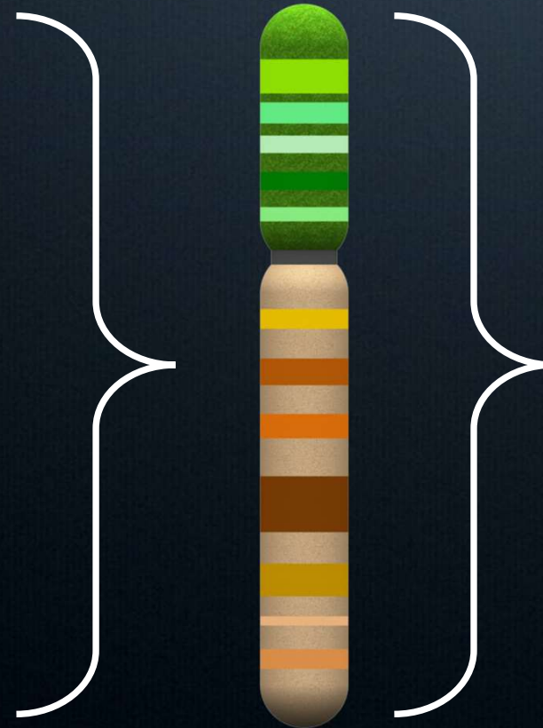
Chromatid
